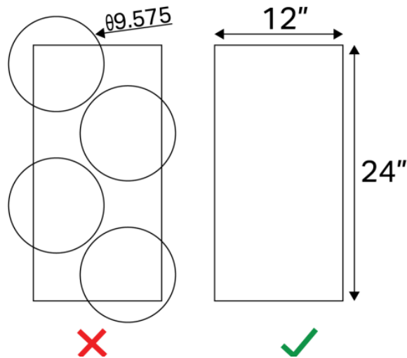
图 35 自制塑料件须可容纳于单块 12" x24" 的塑料板内
