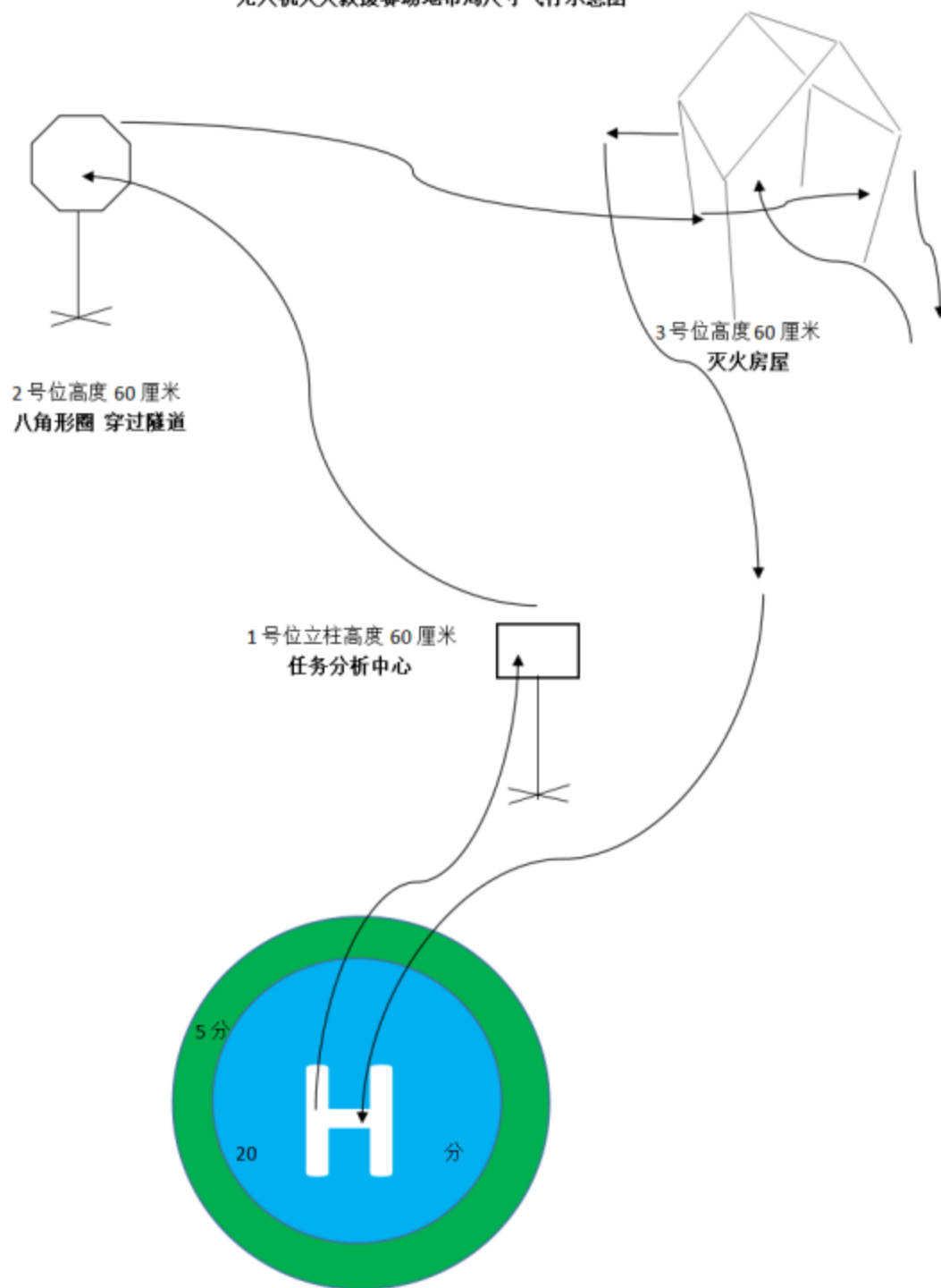
无人机灭火救援赛场地布局尺寸飞行示意图
